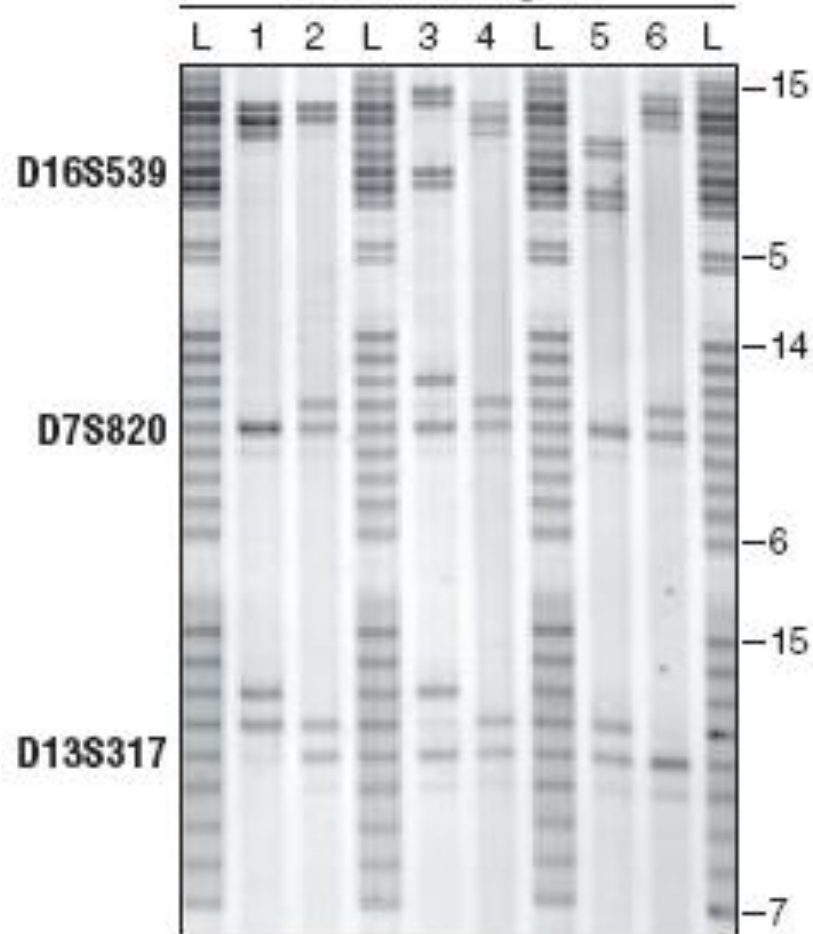
4% Denaturing Gel
